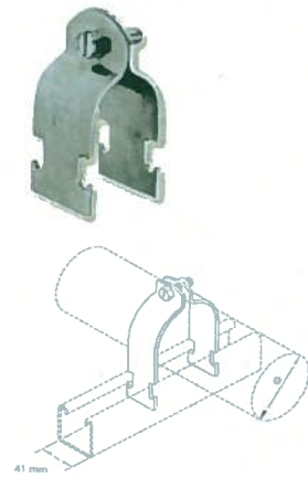
OD Clamp
