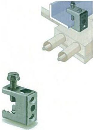
EBC Clamp
