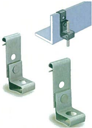
J Clip
